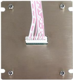
AC-Anschluss (Standard)
